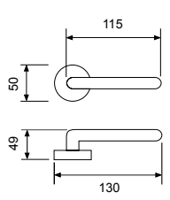
21072R04 - OCL/OCS Handle on rose Maner cu rozeta
